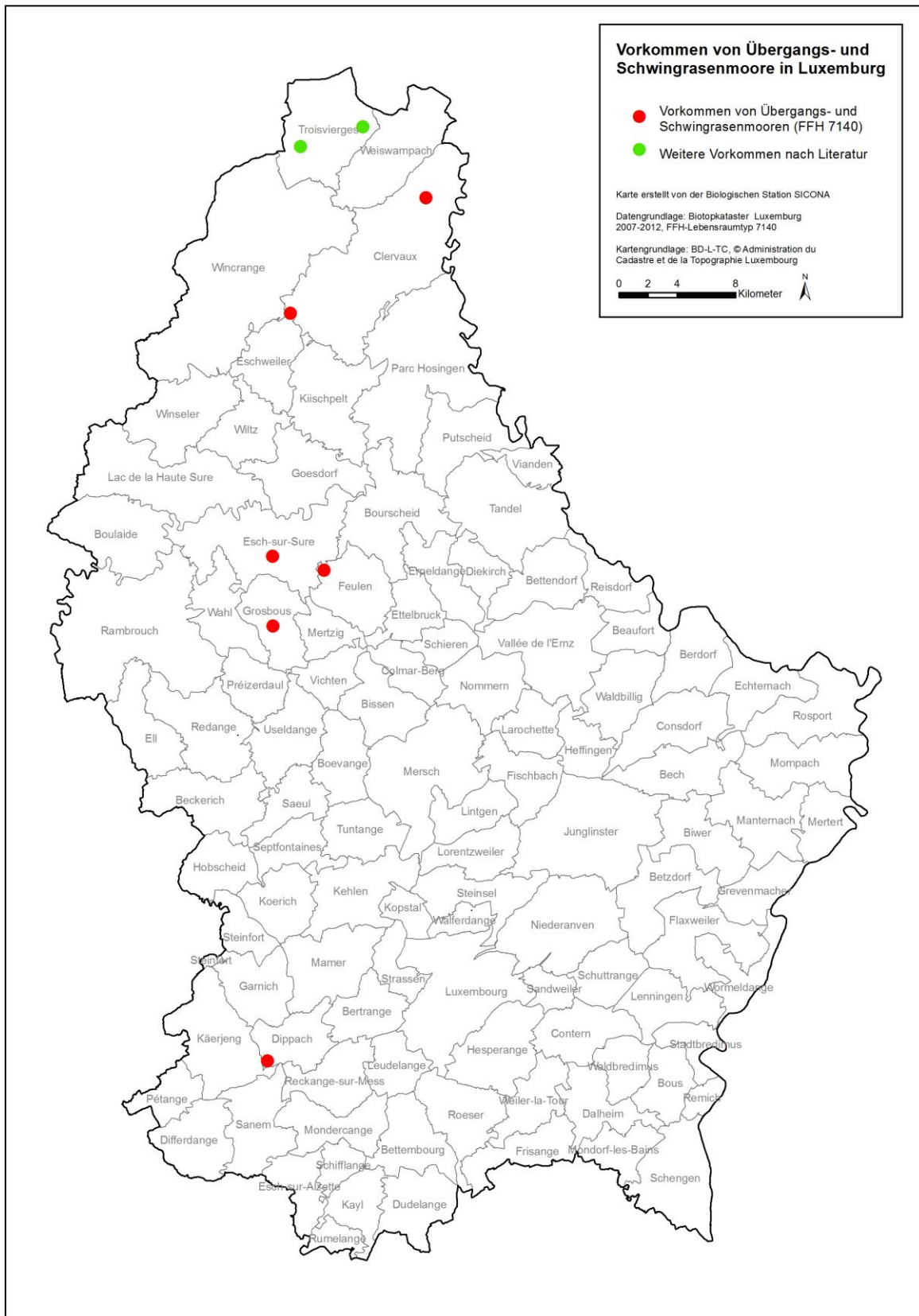
Abb. 1: Verbreitung der Zwischenmoore (FFH7140) in Luxemburg. (Datenbasis: Offenland-Biotopkataster 2013, FFH7140, MINISTÈRE DE L'ENVIRONNEMENT DE LUXEMBOURG 2013 sowie RIES 1993, LANIUS 1995, SCHNEIDER 2011).
